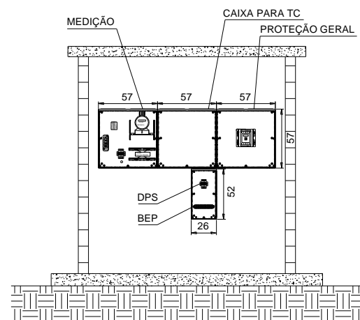
CORTE B-B'
