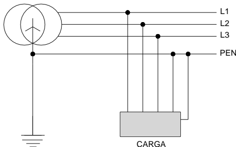
Figura 3 - Esquema TN-C
