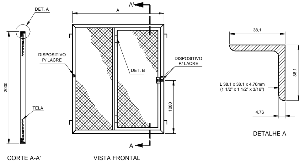
CORTE A-A'
