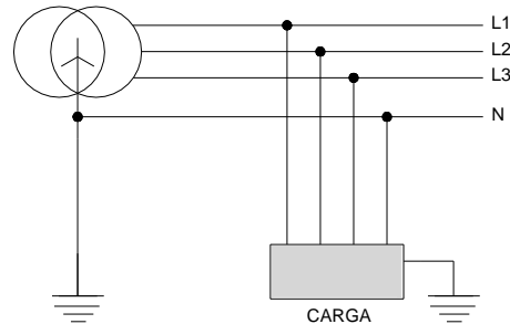
Figura 4 - Esquema TT
