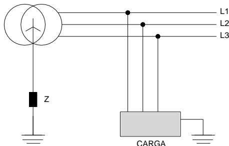
Figura 5 - Esquema IT
